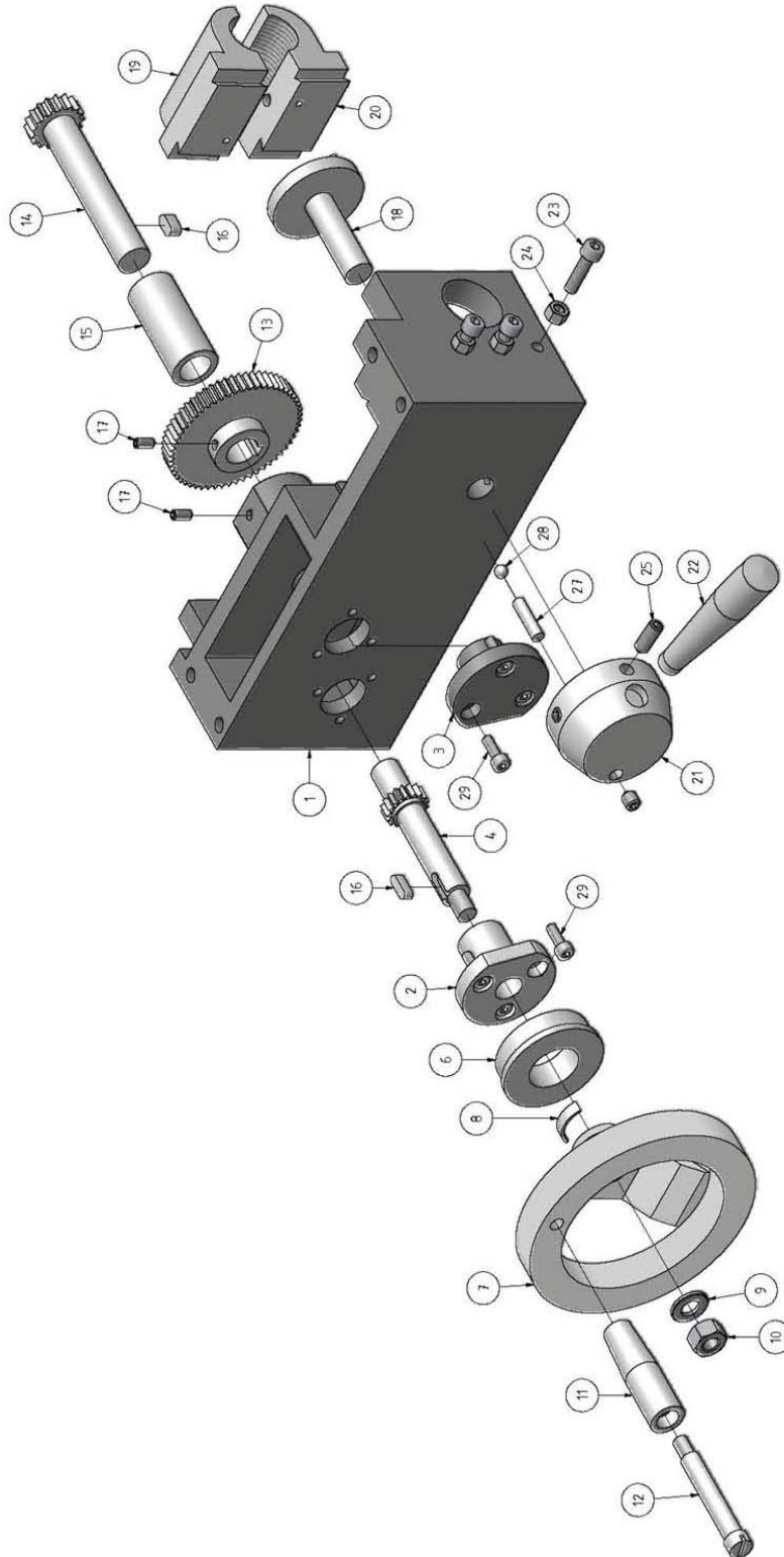
1-4: Bettschlitten - Bed slide
