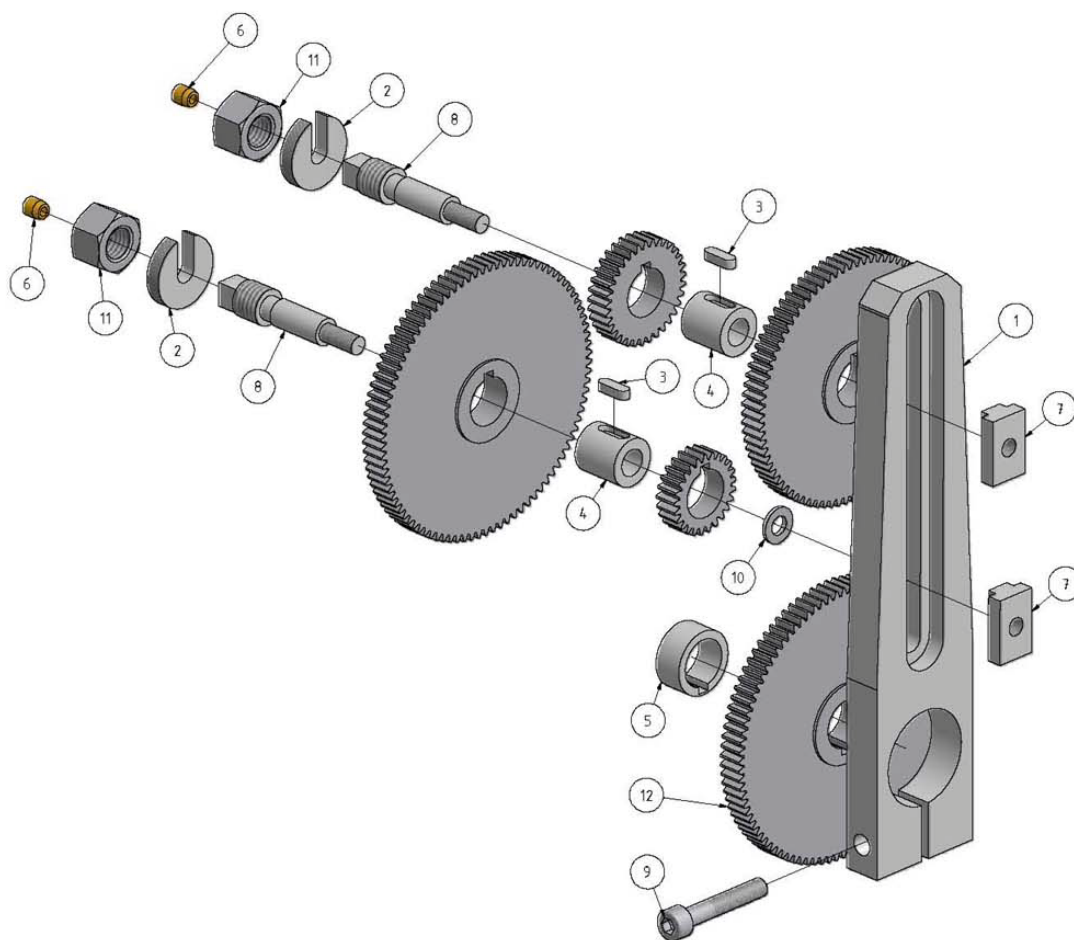
1-3: Wechselradschere
