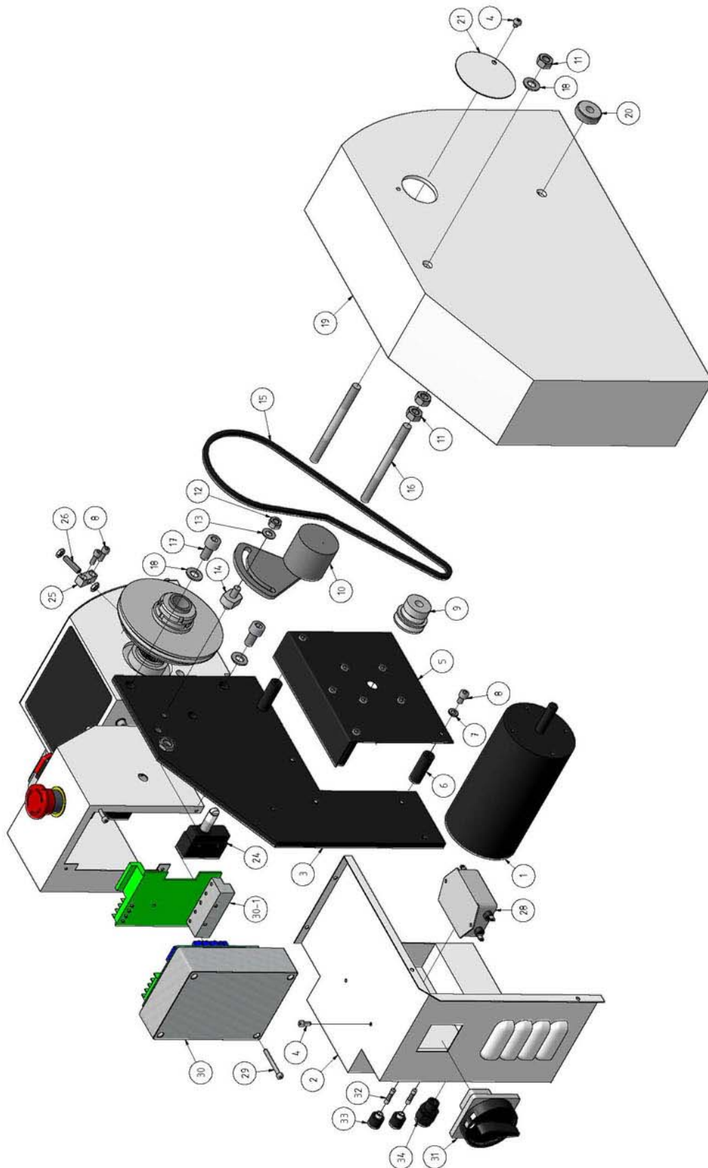
1-10: Vario Antrieb D210 - Vario drive D210
